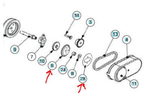
Fig. 1: New Sprocket retainer, pos. 28.
